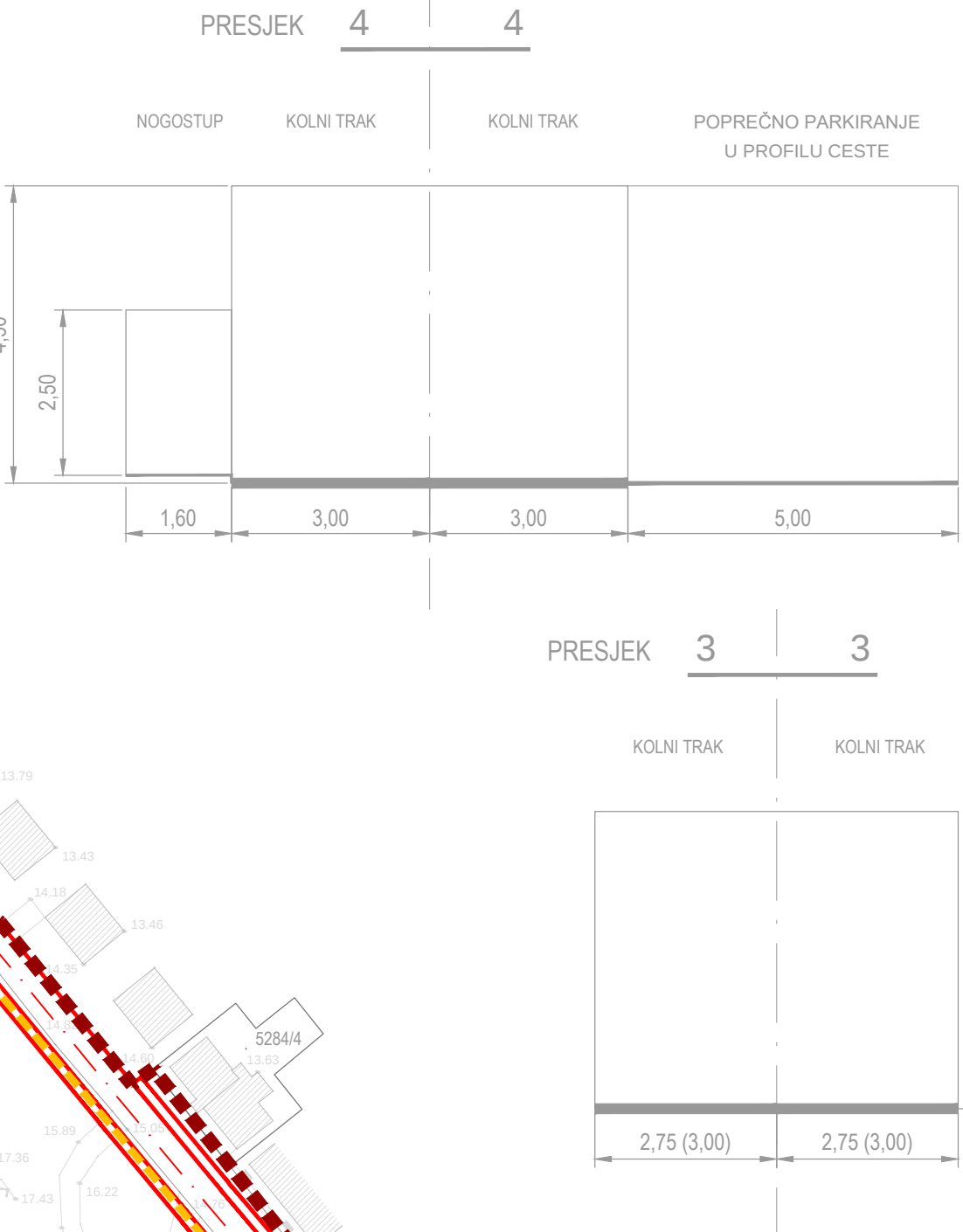
POPREČNI PROFILI 1 :100
