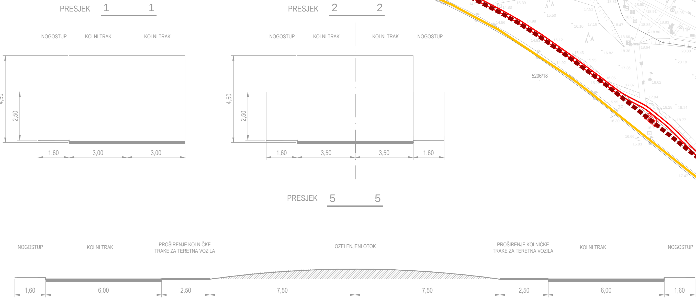
POPREČNI PROFILI 1 :100
