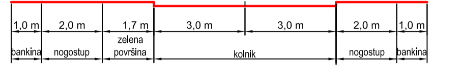
PROFIL 2 - 2
