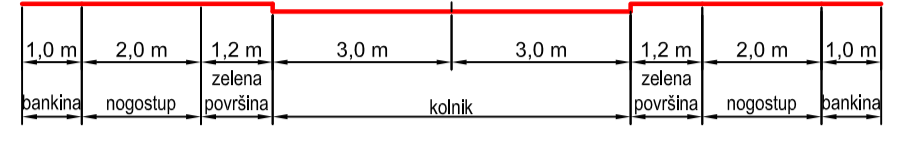
PROFIL 1 - 1
