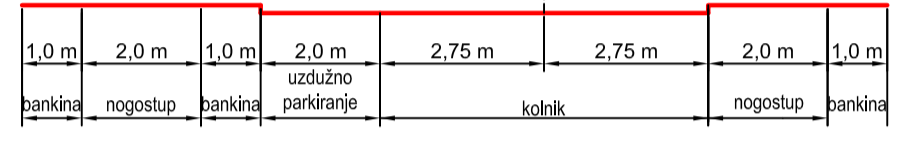
PROFIL 3 - 3
