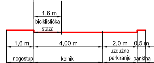
PROFIL 5 - 5
