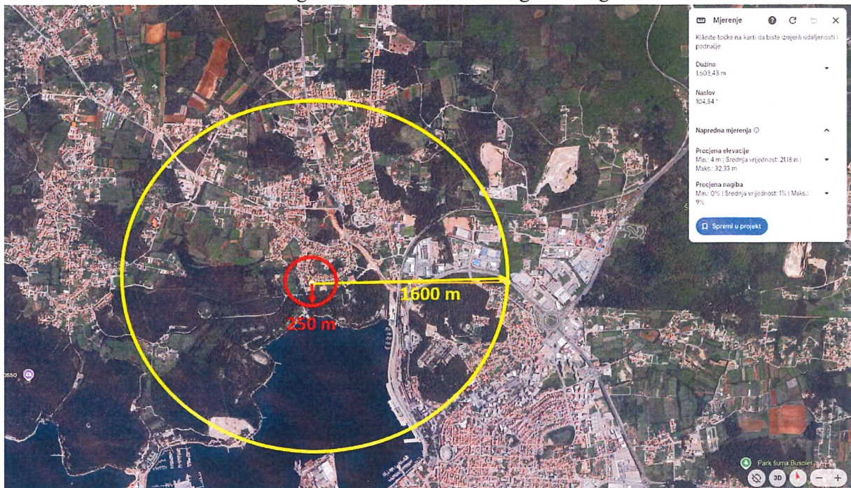
Slika 2. Sigurnosna zona od razlijetanja fragmenata
