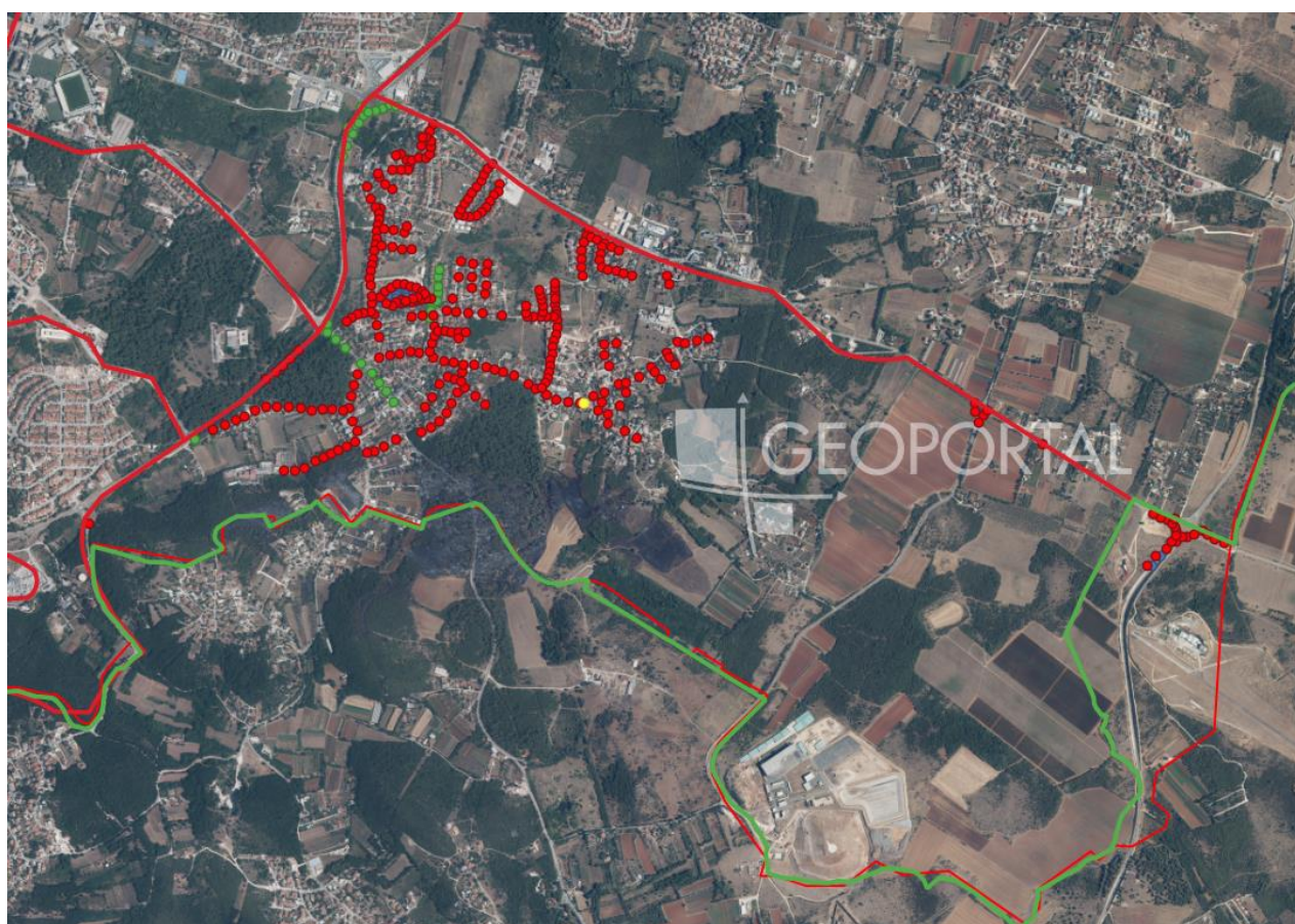
Slika 17. Sustav javne rasvjete na području MO Valdebek
