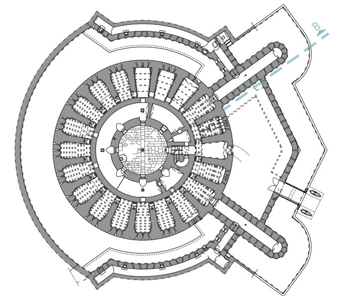
Tlocrt prizemlja
