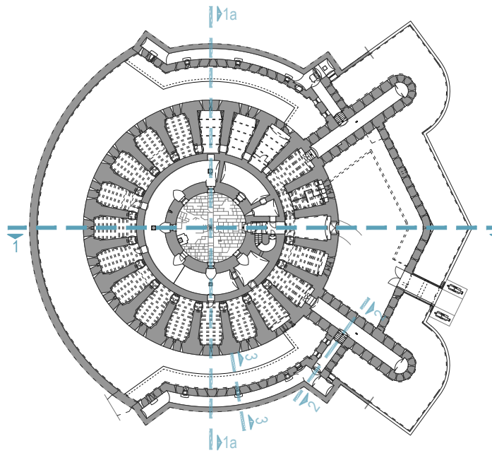
Tlocrt prizemlja
