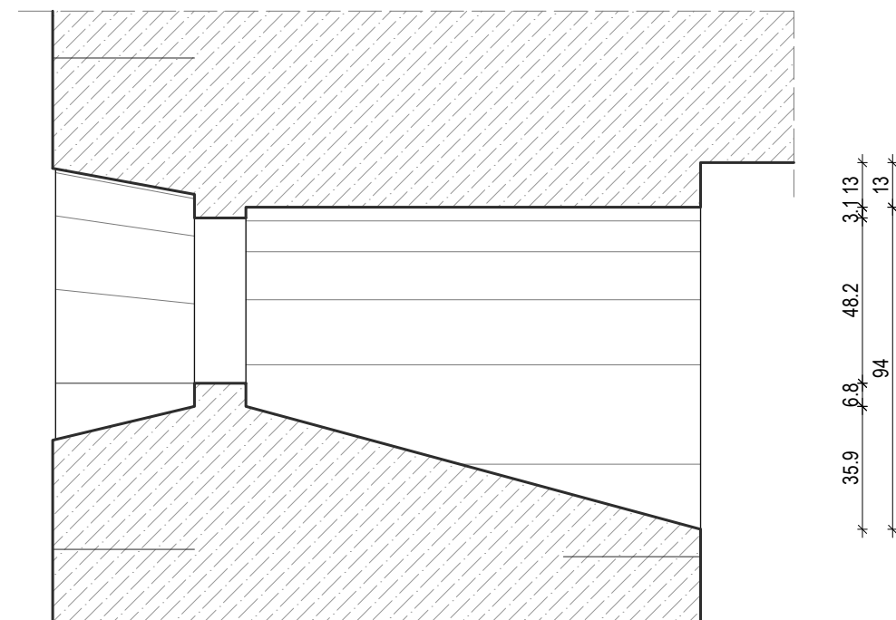
PRESJEK
