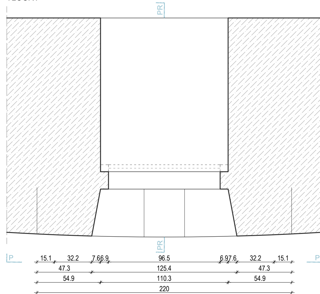
TLOCRT
