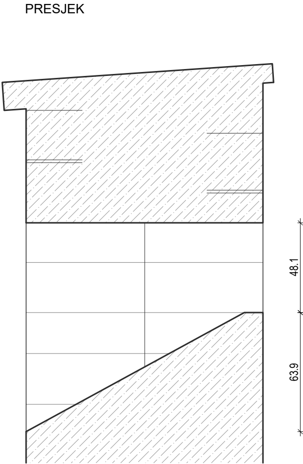
PRESJEK
