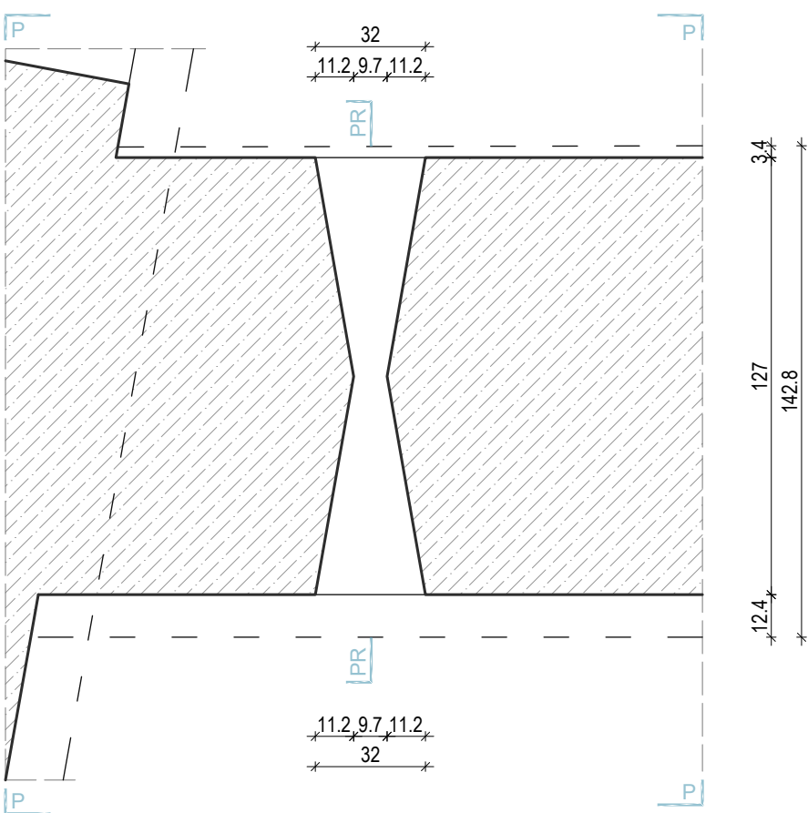
TLOCRT
