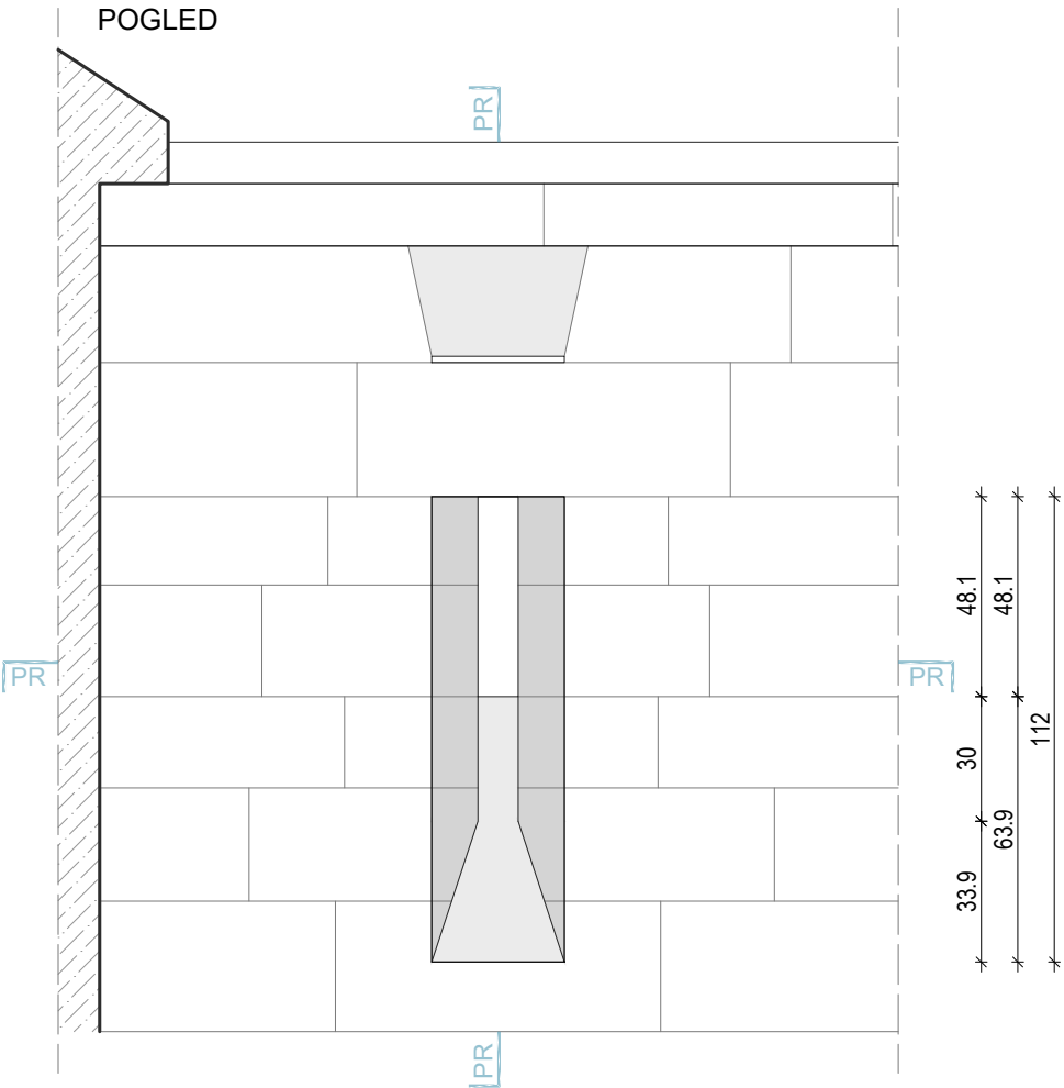
POGLED
