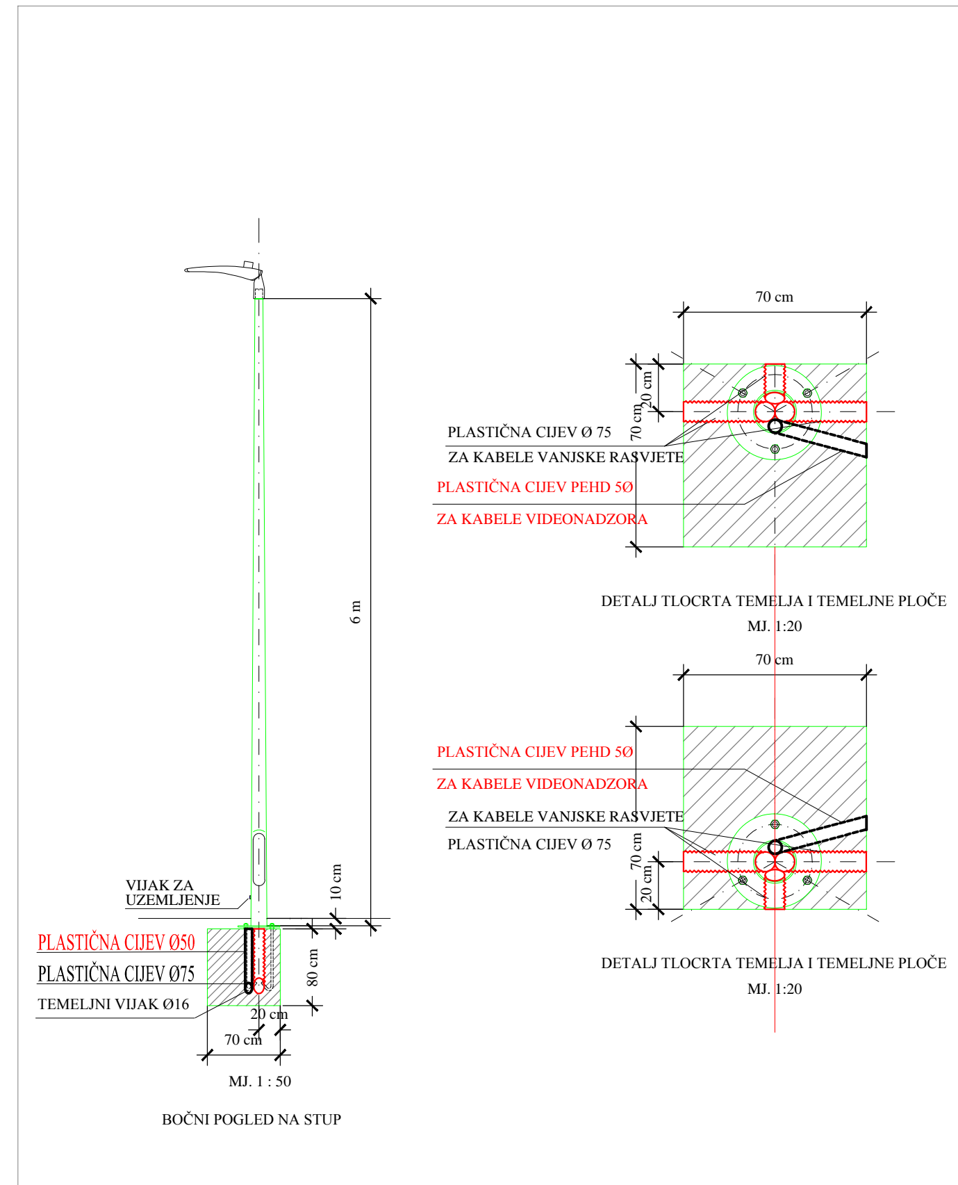
DETALJ UVLAČENJA CIJEVI EKK U RASVJETNI STUP VISINE 6 M
