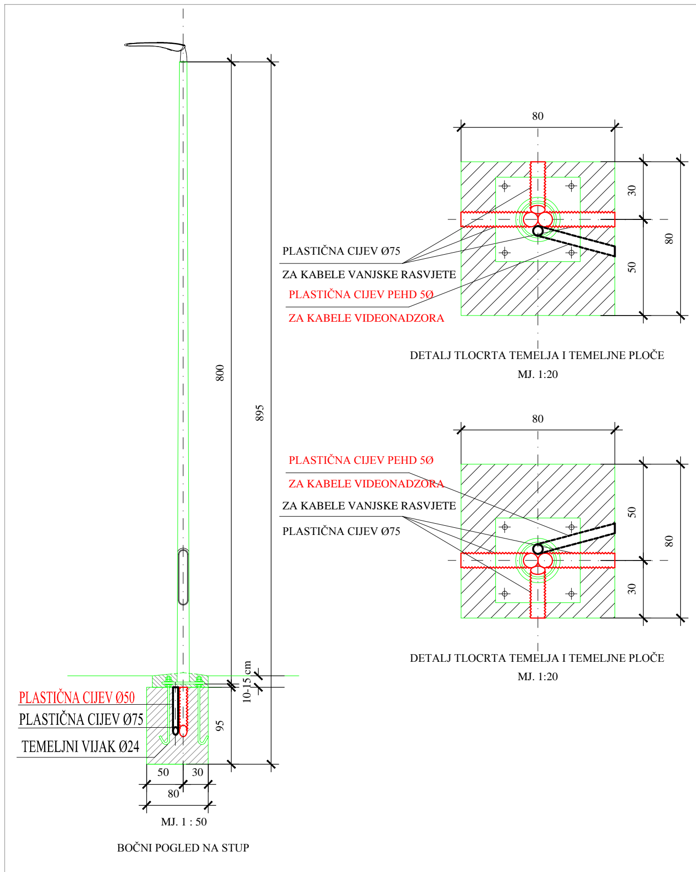
DETALJ UVLAČENJA CIJEVI EKK U RASVJETNI STUP VISINE 8 M
