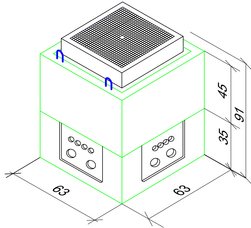
IZGLED ZDENCA MZ D0
