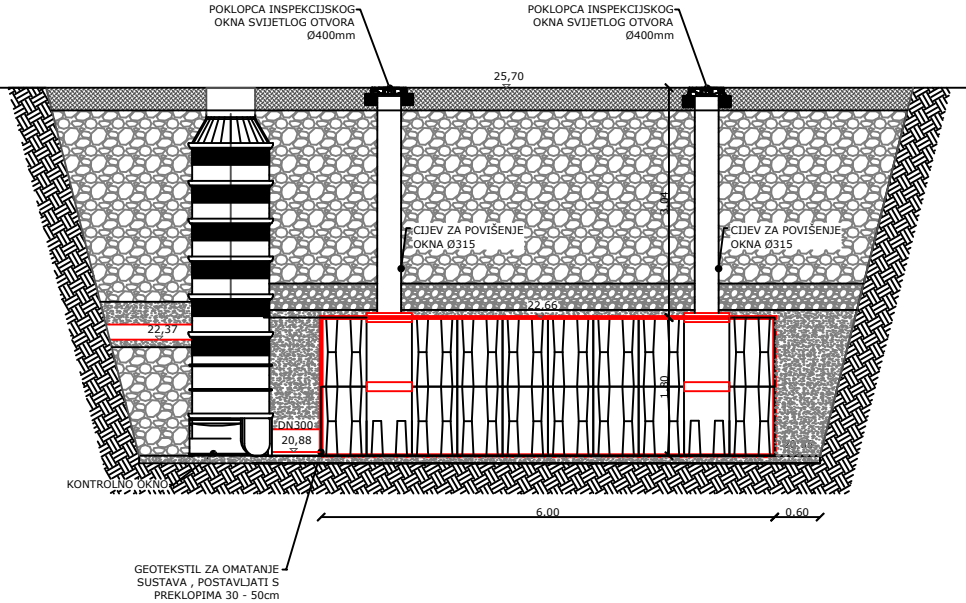
PRESJEK A-A
