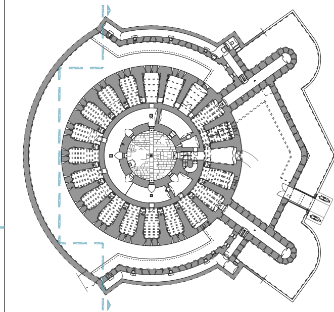
Tlocrt prizemlja
