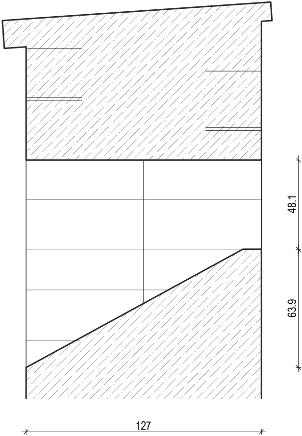
PRESJEK
