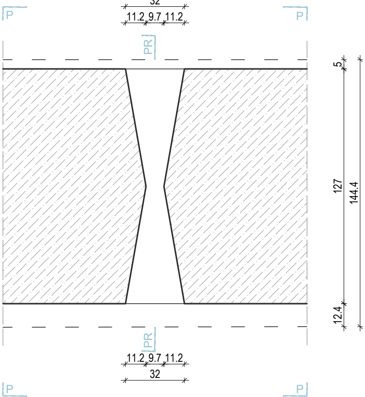
TLOCRT
