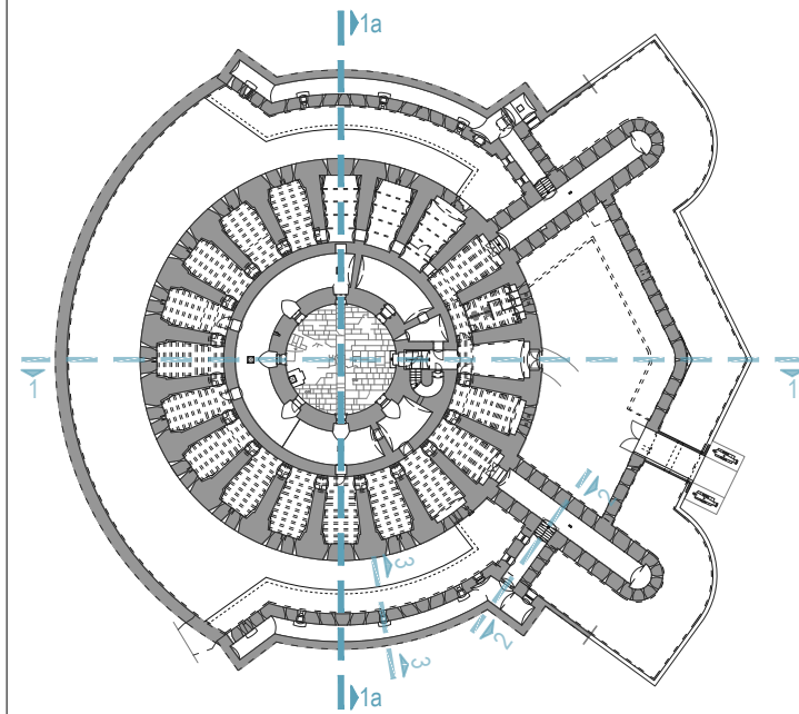
Tlocrt prizemlja
